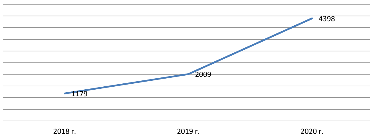
Рисунок 29 Виртуальные справки
